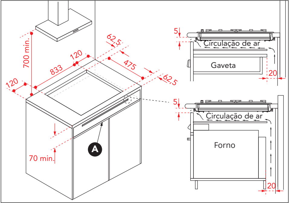
Modelo: CKG-6Q-90-XQ-3ZEB
