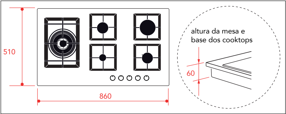
Modelo: CKG-6Q-90-XQ-3ZEB
