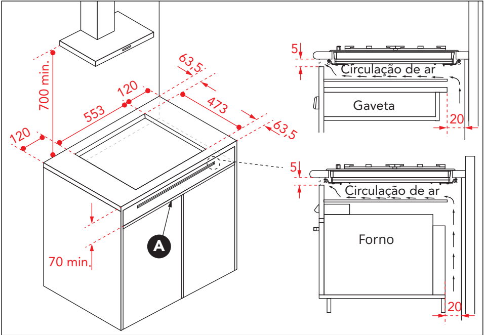
Modelo: CKG-5Q-75-XQ-3ZEA
