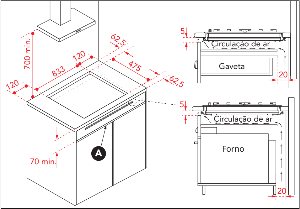
Modelo: CKG-6Q-90-XQ-3ZEB
