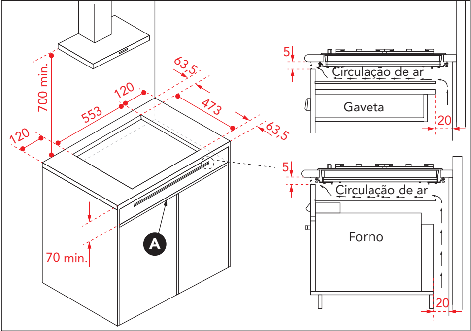
Modelo: CKG-5Q-75-XQ-3ZEA
