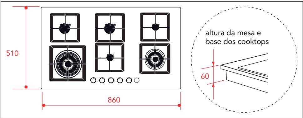
Modelo: CKG-6Q-90-XQ-3ZEB
