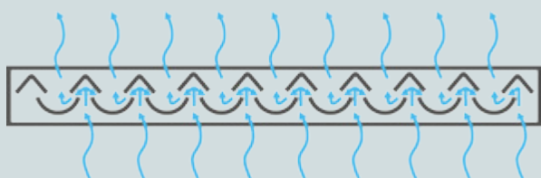
Perfil do filtro com as lâminas entrelaçadas ilustrando a condensação de vapores.
